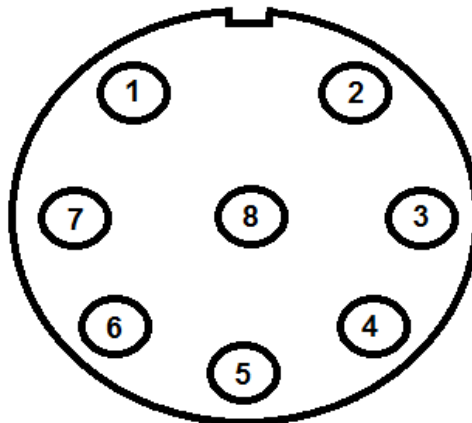
M12 - 8 pin
